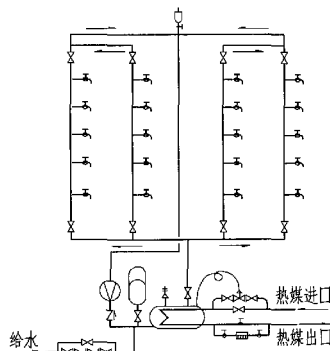
下行上回式循环系统
