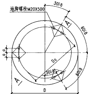
换热器基础
