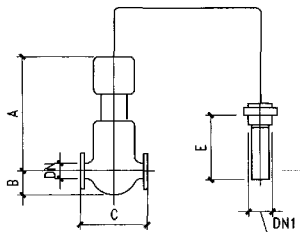
ZWT型自力式温度调节器外形图
