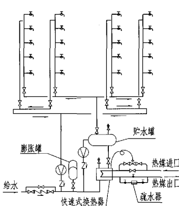
下行下回双立管同程式循环系统
