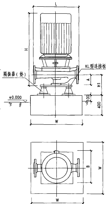
外形及安装
