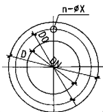
进、出水管道及法兰
