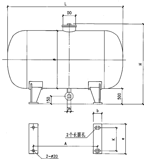
卧式膨胀水罐外形图
